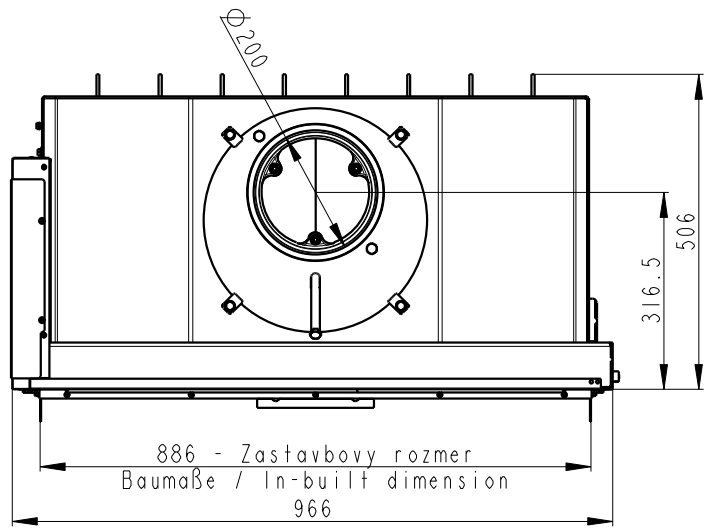
Centralni privod vzduchu Central air inlet Zentralluftzufuhr
