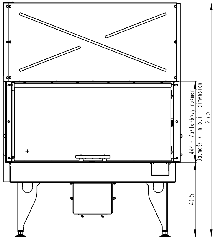
Centralni privod vzduchu Central air inlet Zentralluftzufuhr
